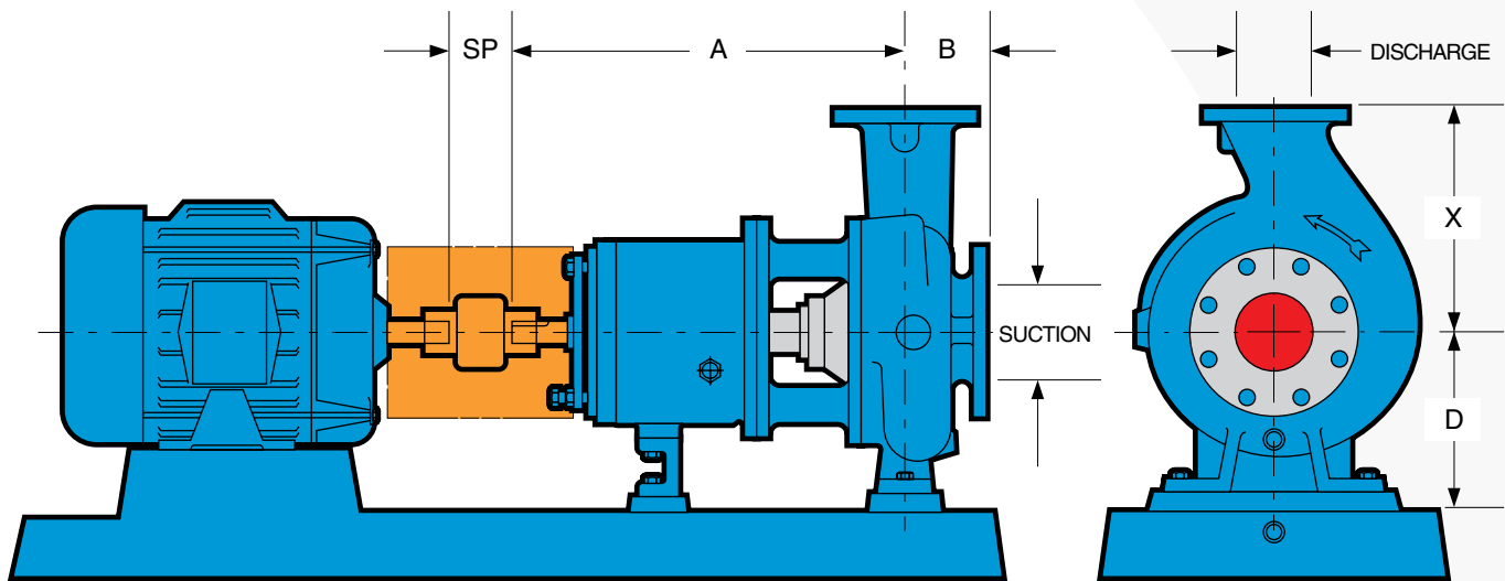
DIMENSIONS
